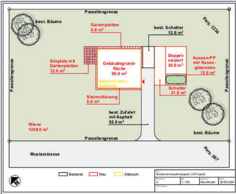
Muster Bodenversieglungsplan 2 (Bauprojekt)
