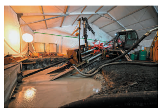
Spülbohrung Titlis
